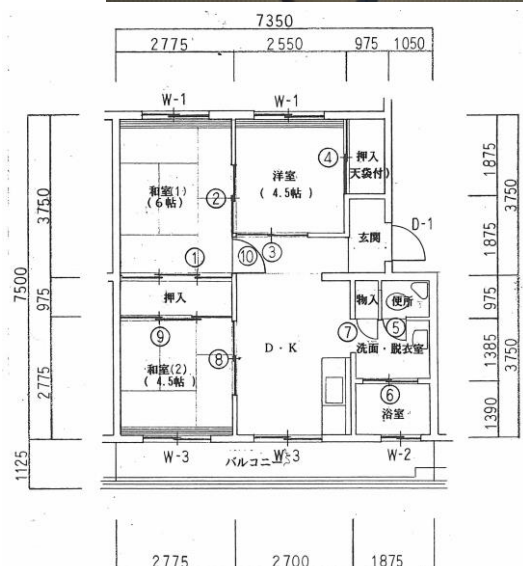
代表間取図（左右反転タイプあり）
