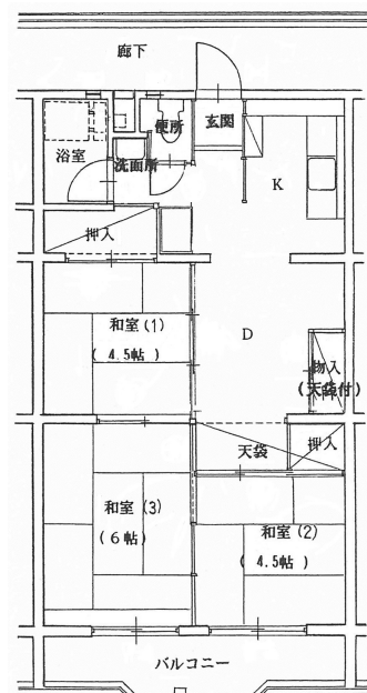
代表間取図（左右反転タイプあり）
