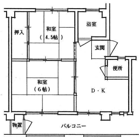
代表間取図（左右反転タイプあり）
