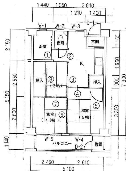
代表間取図（左右反転タイプあり）
