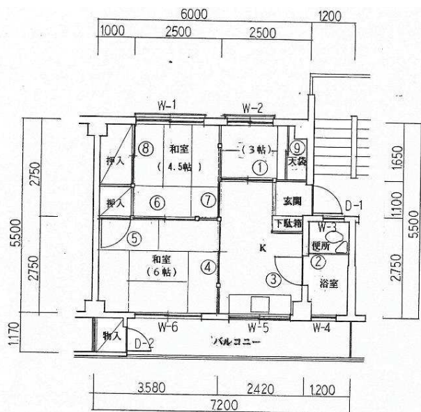
代表間取図（左右反転タイプあり）
