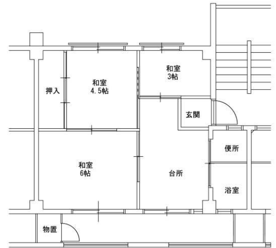
代表間取図（左右反転タイプあり）
